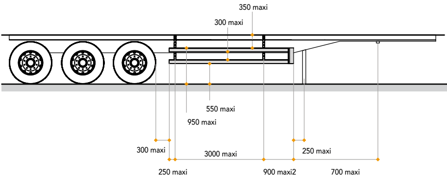
SEMIREMOLQUE CLASE 03 Y 04
