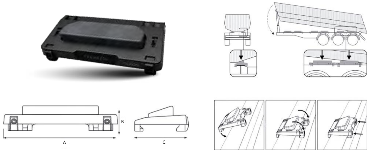
ALMOHADILLA SOPORTE VOLCADO
