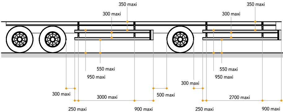
REMOLQUE CLASE 03 Y 04
